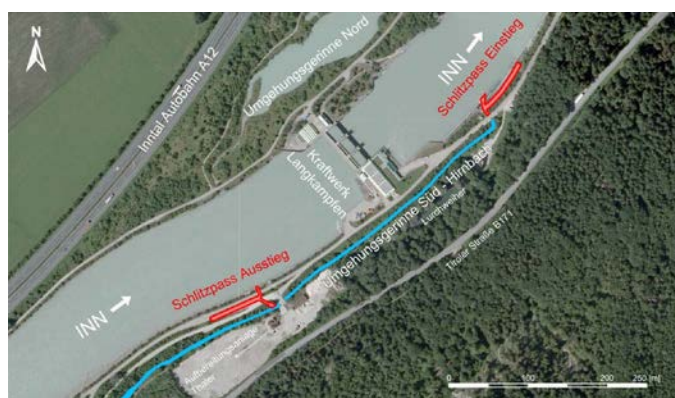
Neue Fischwanderhilfe für das Kraftwerk Langkampfen.
